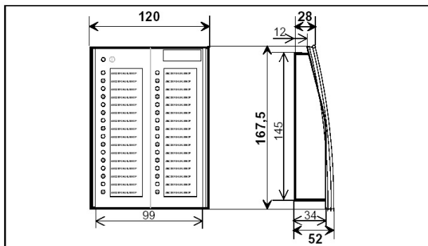
Рис. 2 Габариты PIM 731 и FGG 716 (в мм)
