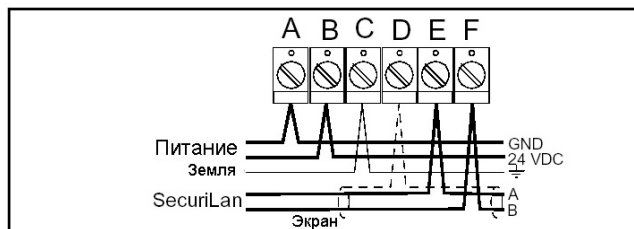
Рис. 4 Подключение PIM 731
