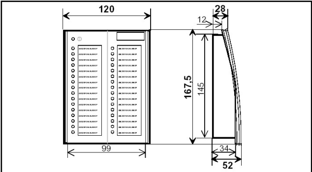
Рис. 2 Габариты pIM 732 и FG 716 (в мм)
