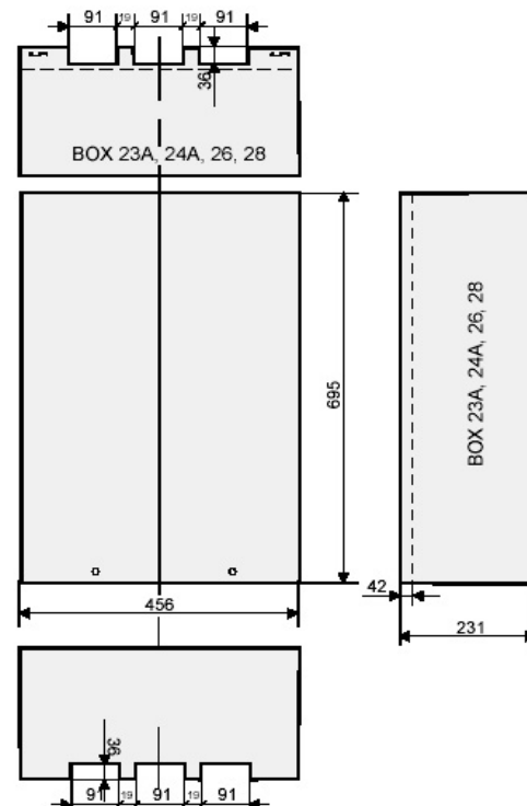
Рис. 4 Габариты MCU 211B
