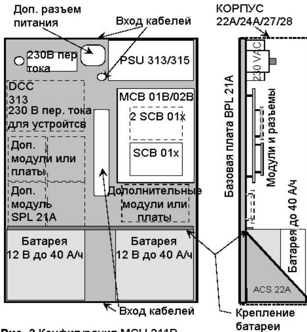
Рис. 2 Конфигурация MCU 211B
